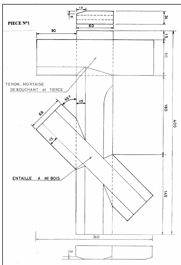
FICHE DE DEBIT
